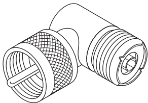
200-197 UG644/U
