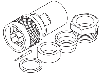
200-720 RG8A/11 UG21B/U
