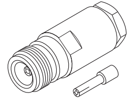
200-726 RG8A/11 UG23E/U
