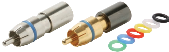
200-085 RG6 RCA – Gold 200-067 RG6 RCA – Nickel 200-083 RG59 RCA – Gold 200-068 RG59 RCA – Nickel 200-081 Mini RG59 RCA – Gold 200-069 Mini RG59 RCA – Nickel 200-087 RG6-Quad RCA – Gold 200-070 RG6-Quad RCA – Nickel
