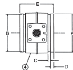
GD-6765-8N Grooved 2½", 3", 4", 6", 8", 10"
