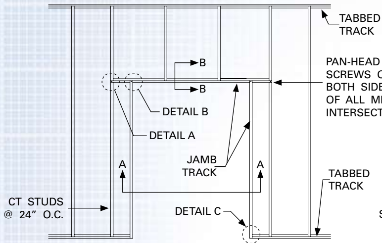
1 DOOR FRAME ELEVATION
