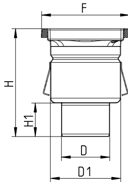
Bottom Outlet
