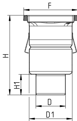
Bottom Outlet
