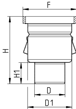
Bottom Outlet
