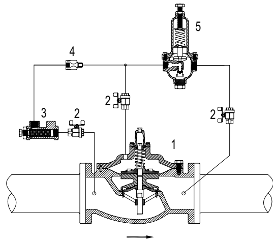
Schematic A-10159B UL
