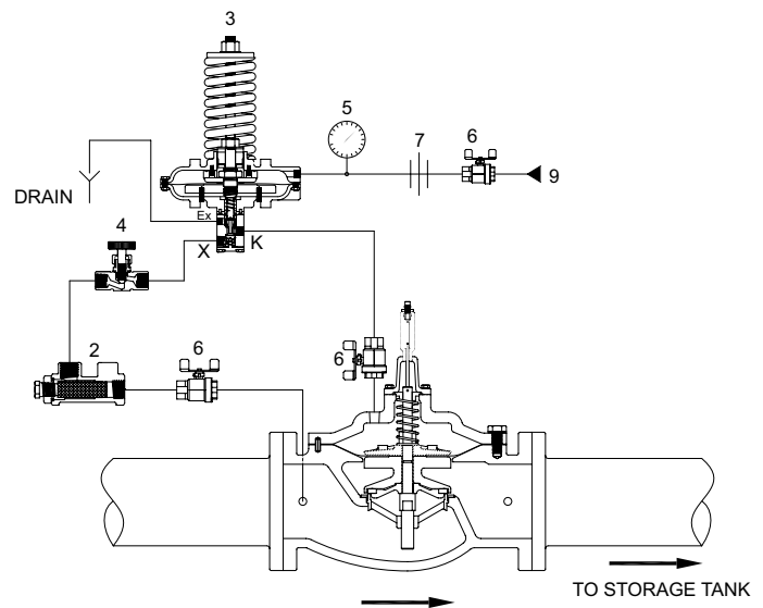
Schematic A-0413C
