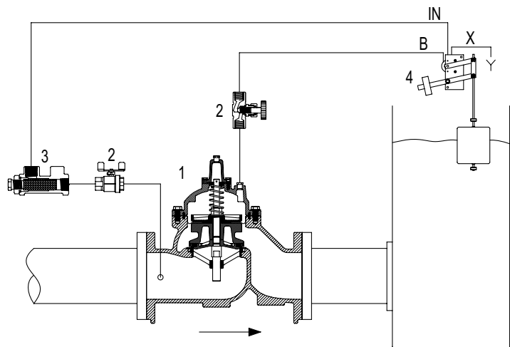
Schematic A-0421C
