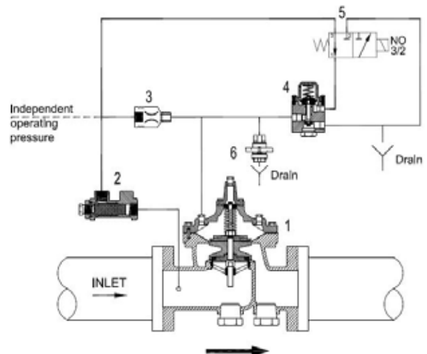
Schematic A-10507A
