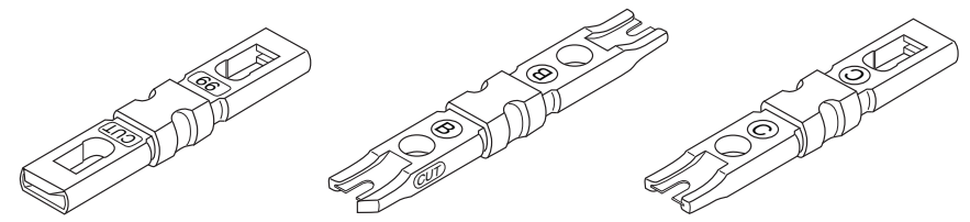
300-670 Type 66 300-675 Type 110/88 300-680 Type 66 110/88
