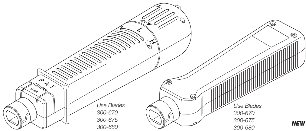
300-650 Adjustable Impact Use Blades 300-670 300-675 300-680 300-655 Non-Adjustable Impact Use Blades 300-670 300-675 300-680 300-656 Non-Impact
