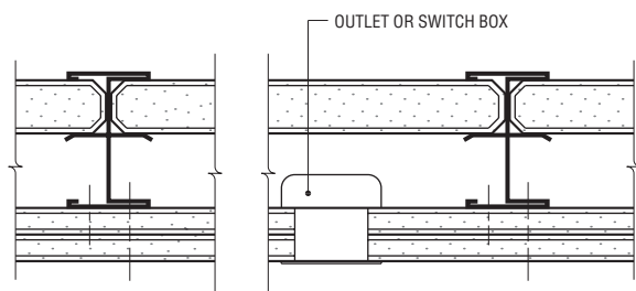
CROSS SECTION 09260V Scale: 3" = 1'-0"
