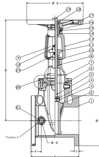
F-607-RWS Flg x Flg
