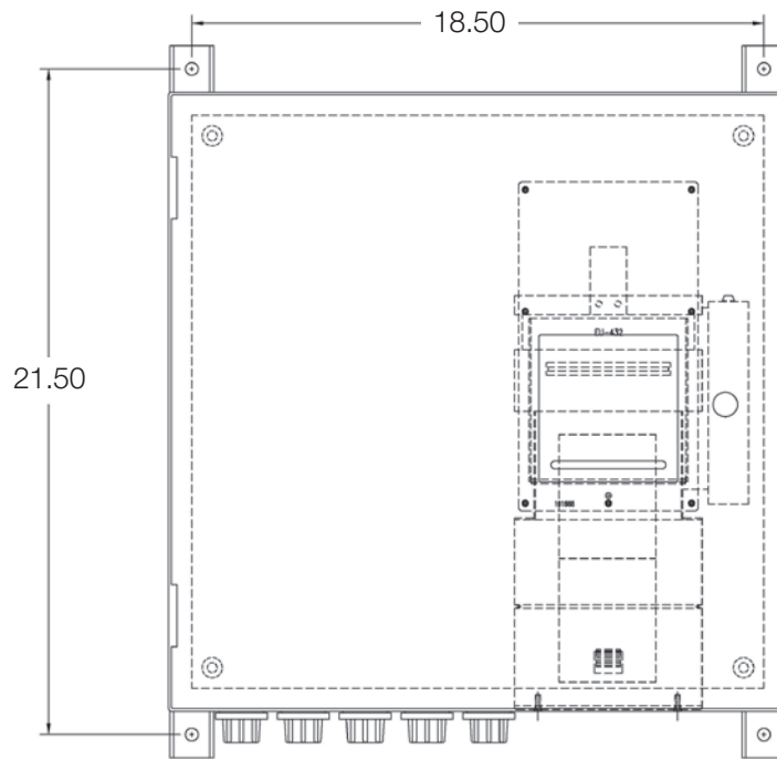
Printer Kiosk
