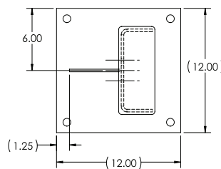
PN 156532 photo eye stand kit dimensions
