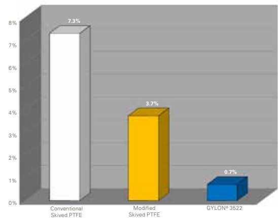
% Void Content
